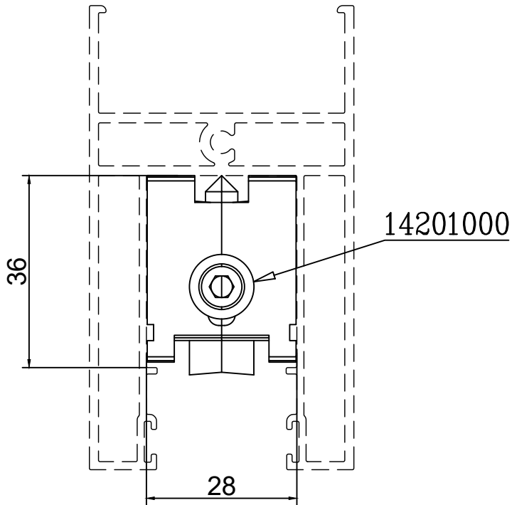
כנף תחתון להרכבת גלגל HD
