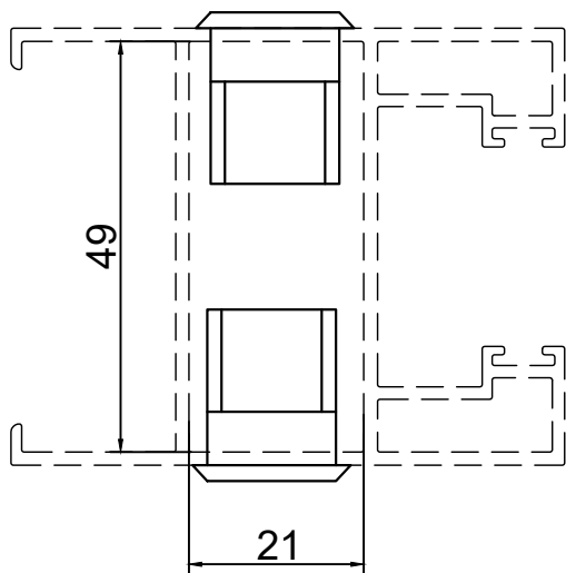
כנף צד להרכבת סגר
