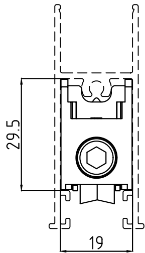
כנף תחתון להרכבת גלגל
