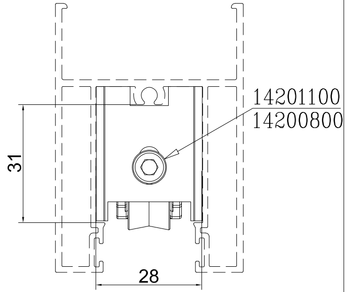
כנף תחתון להרכבת גלגל
