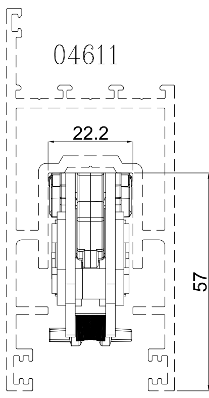
04611 כנף לזיגוג עד 30 מ"מ - משקל עד: 300kg/400kg
