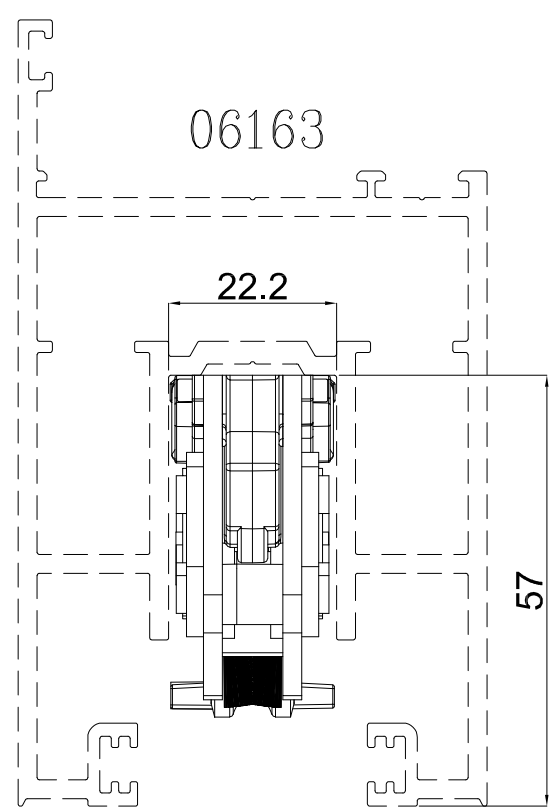
06163 כנף לזיגוג עד 47 מ"מ עם צילון - משקל עד: 300kg/400kg
