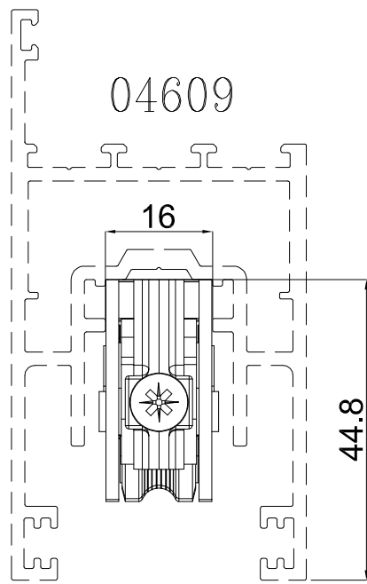
04609 כנף לזיגוג עד 30 מ"מ - משקל עד: 200kg
